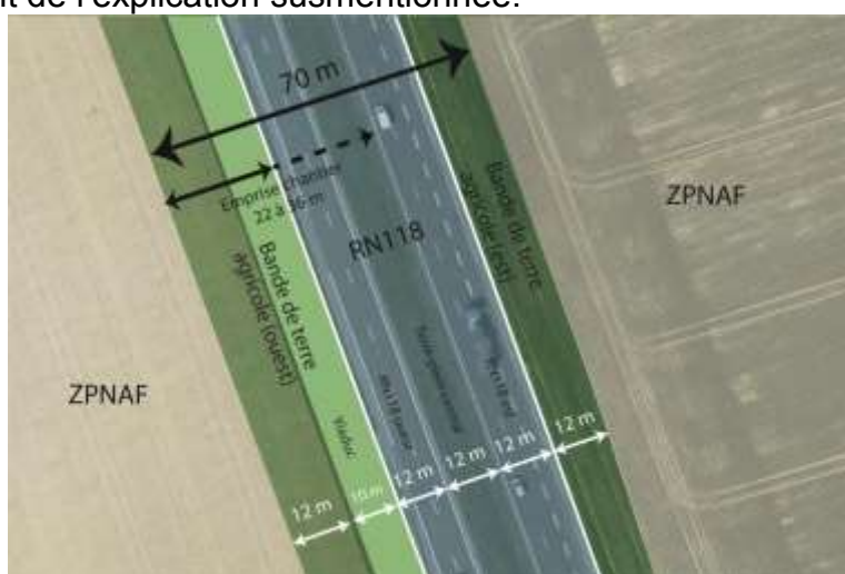
Schéma de principe de l'emprise chantier le long de la RN118 (annule et remplace le schéma de la page 54 du mémoire en réponse ci-dessus)
