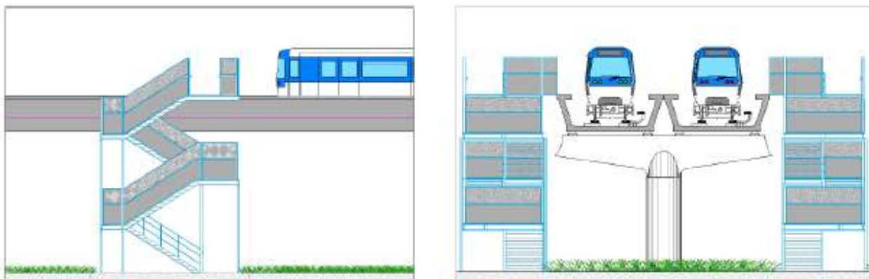
Escaliers de secours – profil en long et coupe (Société du Grand Paris)
